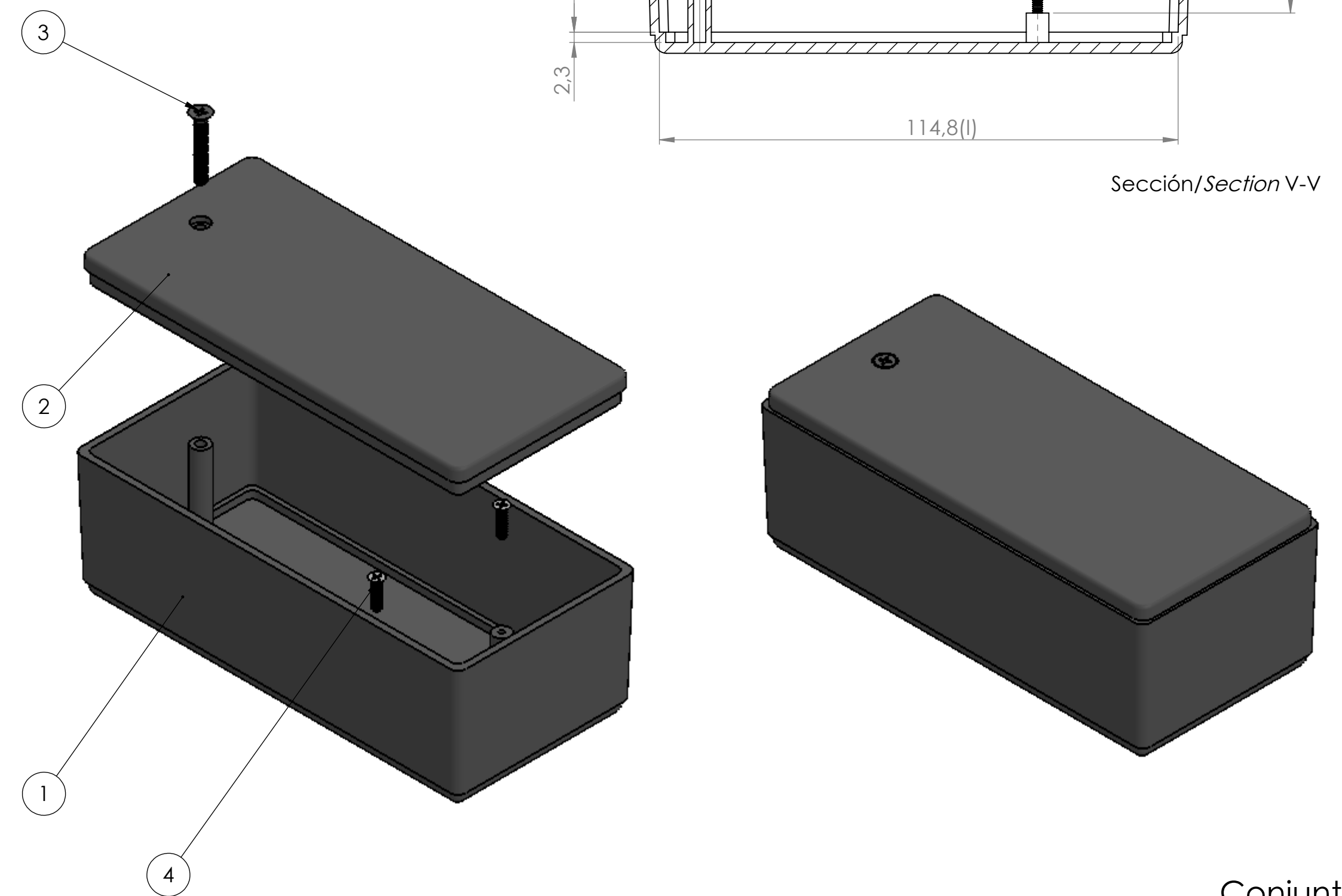
Conjunto Assembly
