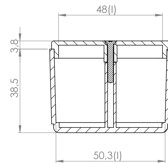
Sección/Section U-U
