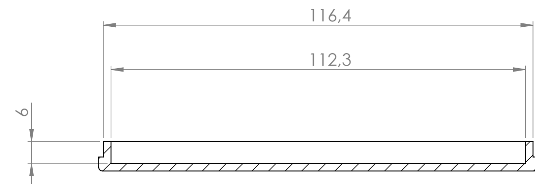
Sección/Section X-X
