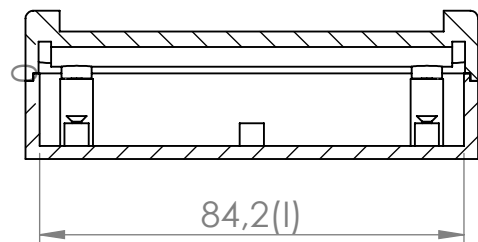
Sección / Section P-P
